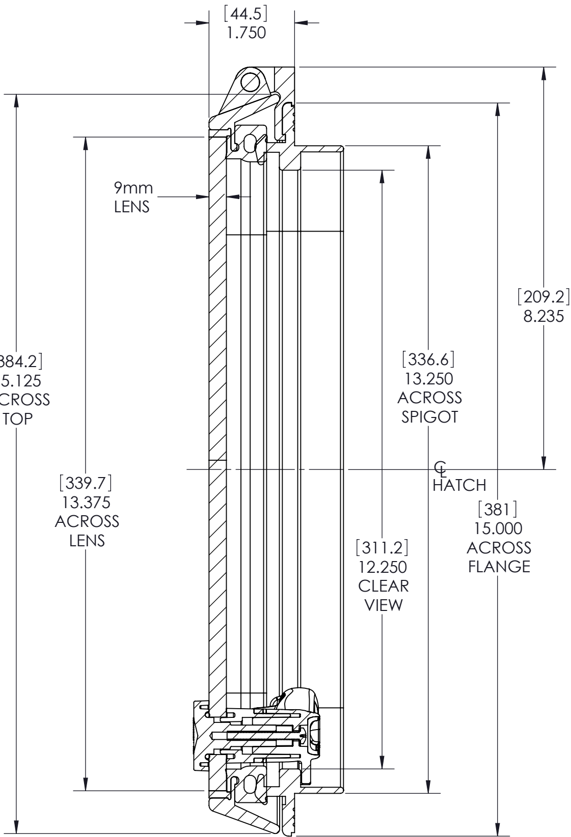
SECTION A-A
